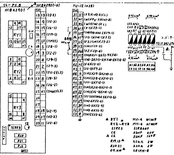
1. 系統図 HCS31572
