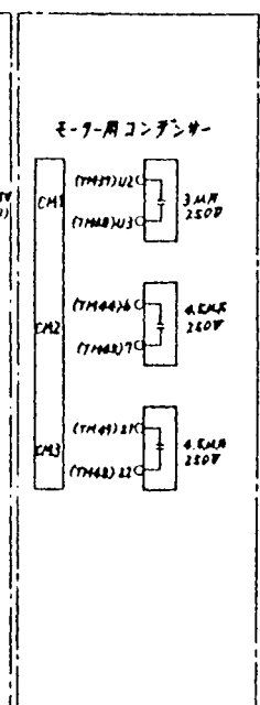
1. 系統図 HCS31572
