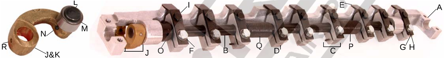
GRIPPER BAR ASSEMBLY - GTO 46 / 52
